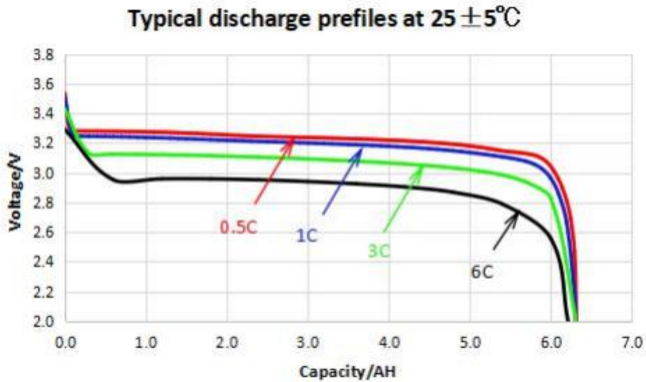
6.0Ah 磷酸铁锂系电池不同倍率放电曲线 Different rate discharge curve of 6.0Ah LiFePO 4 cell
